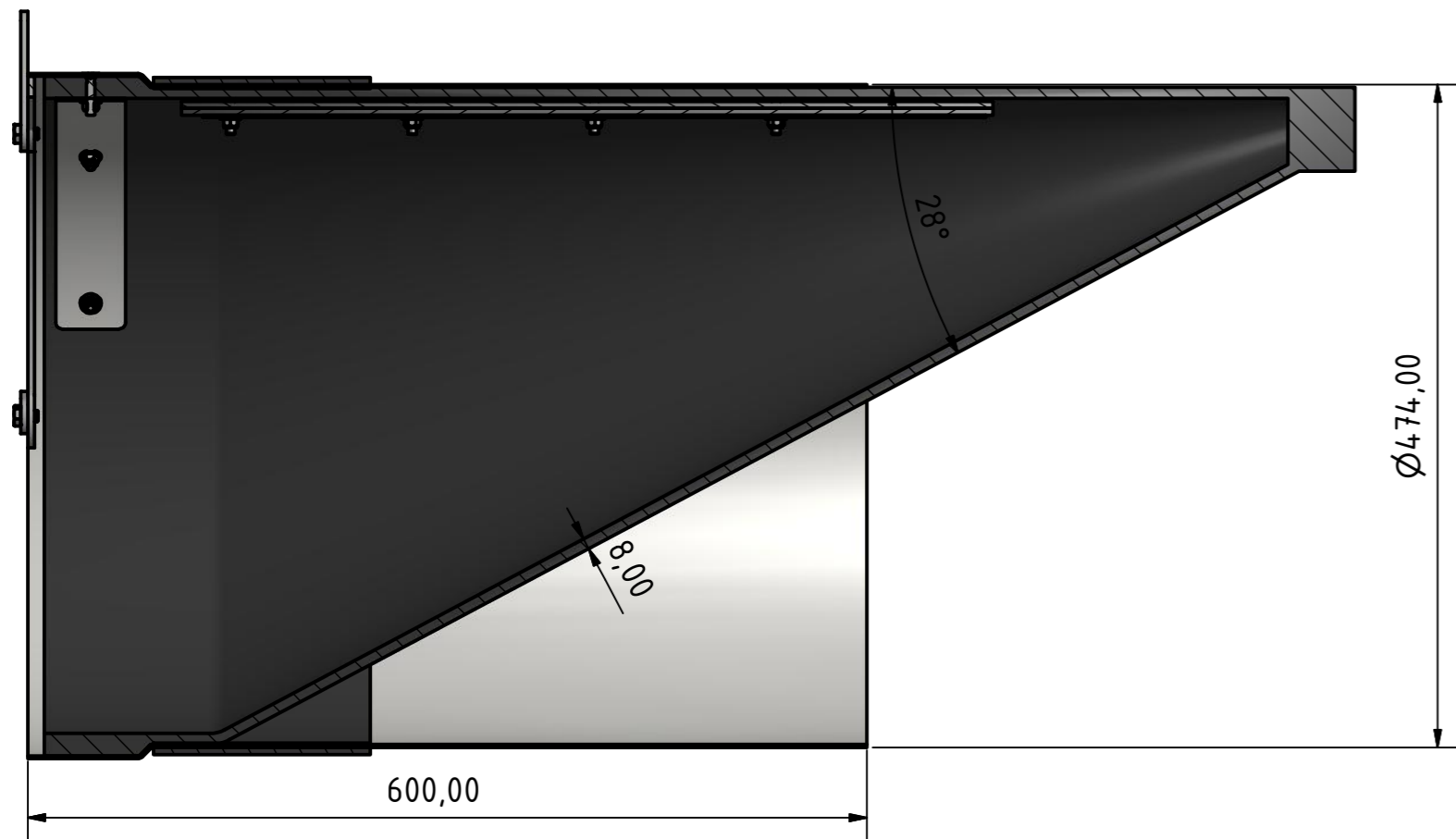
A-A ( 1 : 5 )
